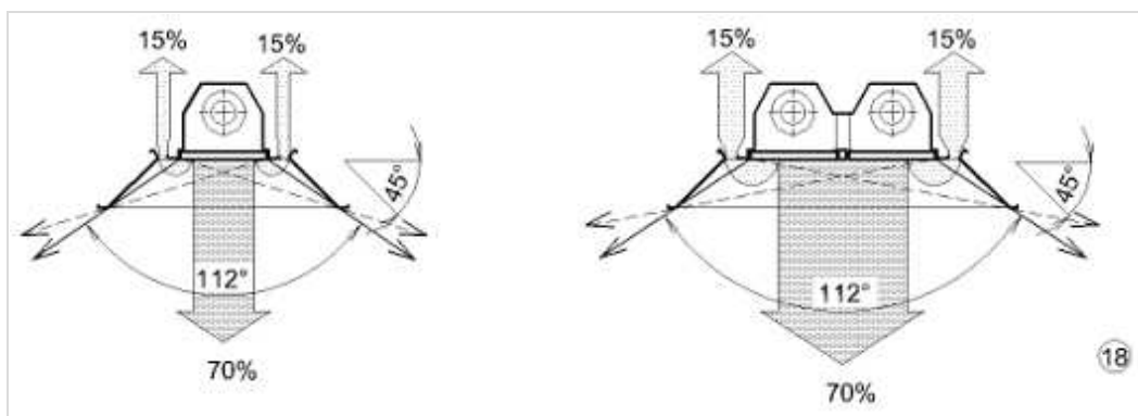
Obr. 18 - Světlé zářiče vodorovné MKV B (beta) jednořadé, resp. dvouřadé
