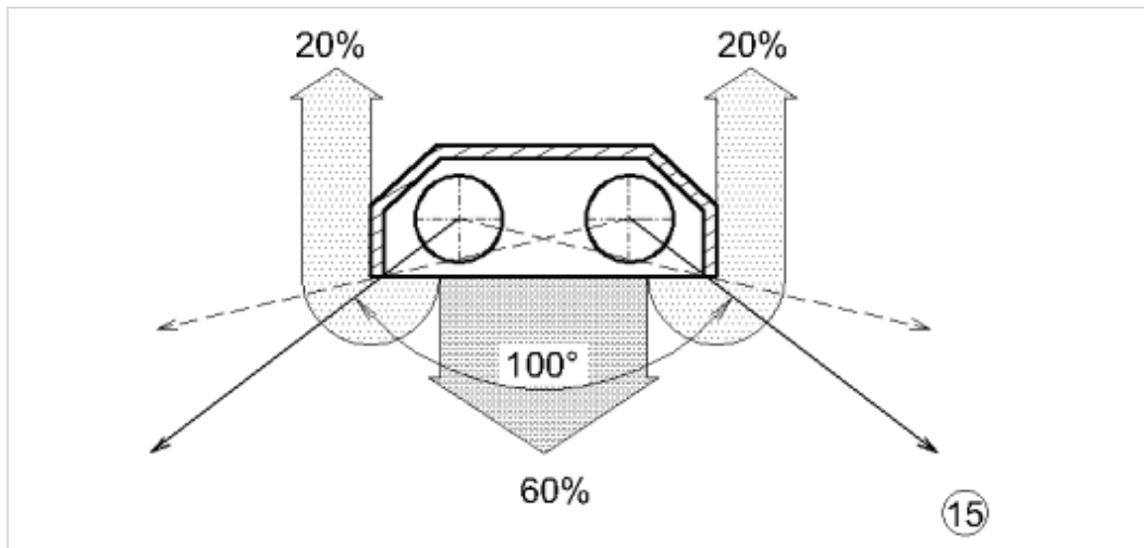
Obr. 15 - Kompaktní zářič v řezu
