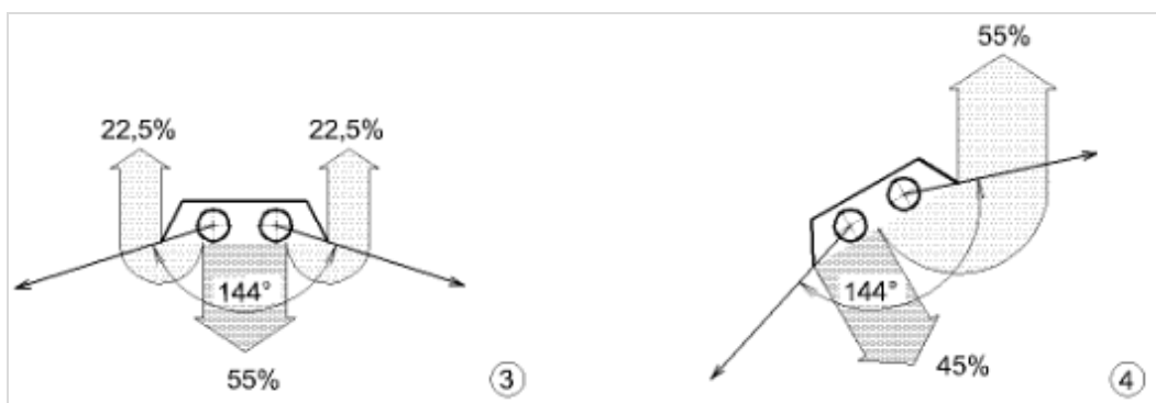
Obr. 3, 4 - Tmavý zářič s mělkým jednoduchým zákrytem a bez koncových čel vodorovný a zavěšený šikmo
