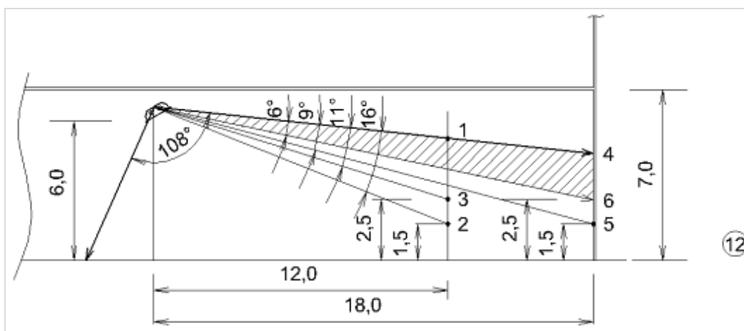
Obr. 12 - Ztrátová složka sálání při naklonění zářiče KMU alfa 30°
