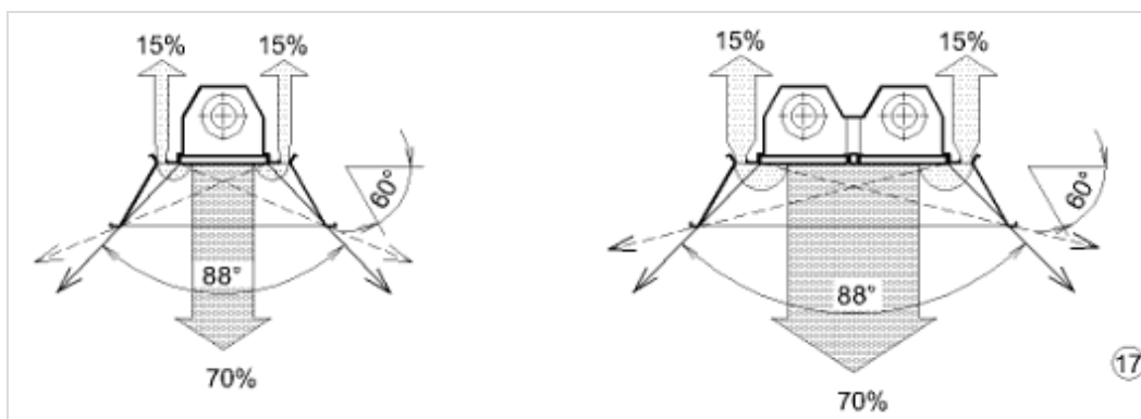
Obr. 17 - Světlé zářiče vodorovné MKV A (alfa) jednořadé, resp. dvouřadé
