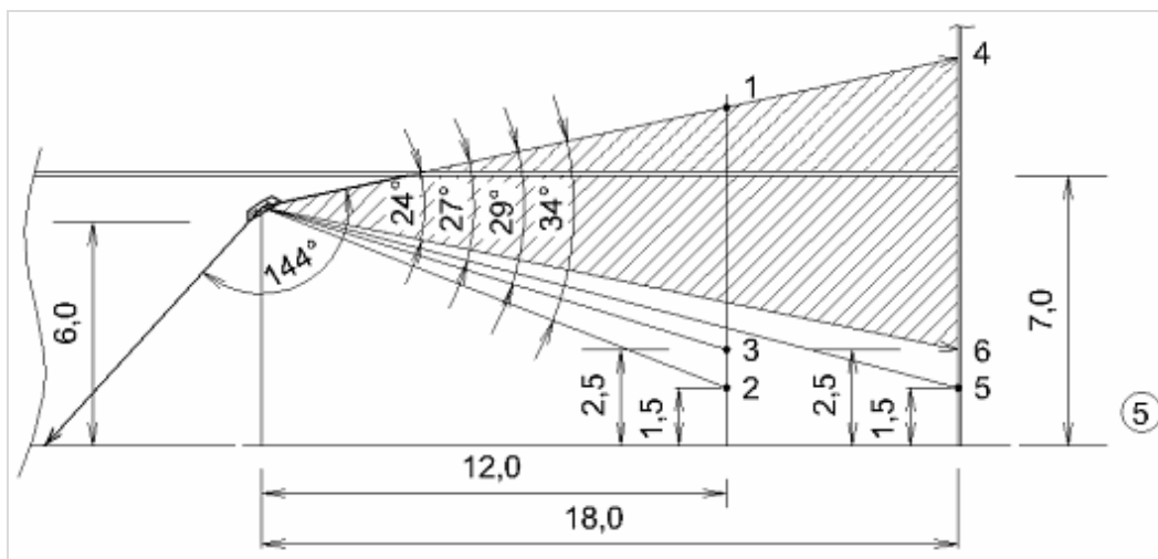
Obr. 5 - Ztrátová složka sálání při naklonění mělkého zářiče 30°
