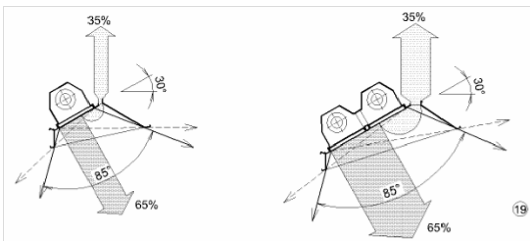
Obr. 19 - Světelné zářiče šikmé MKS jednořadé, resp. dvouřadé
