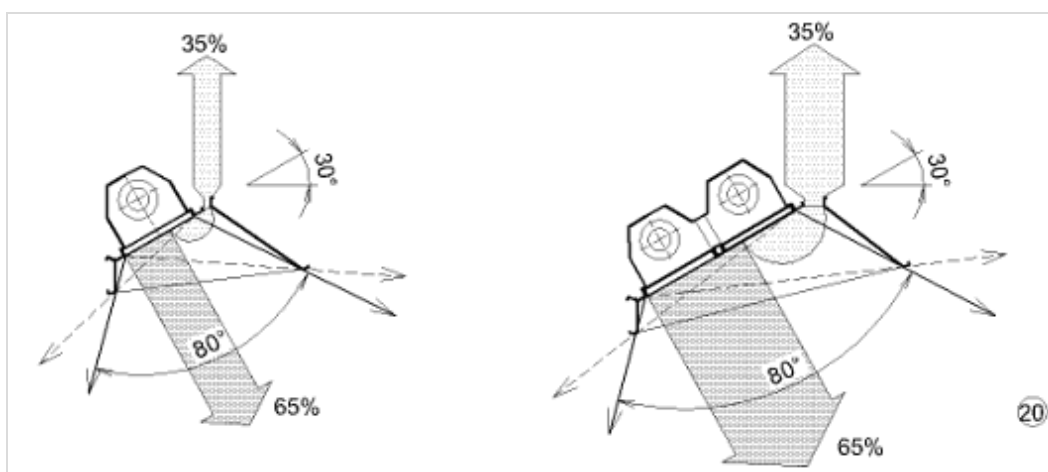
Obr. 20 - Světelné zářiče šikmé MKP jednořadé, resp. dvouřadé
