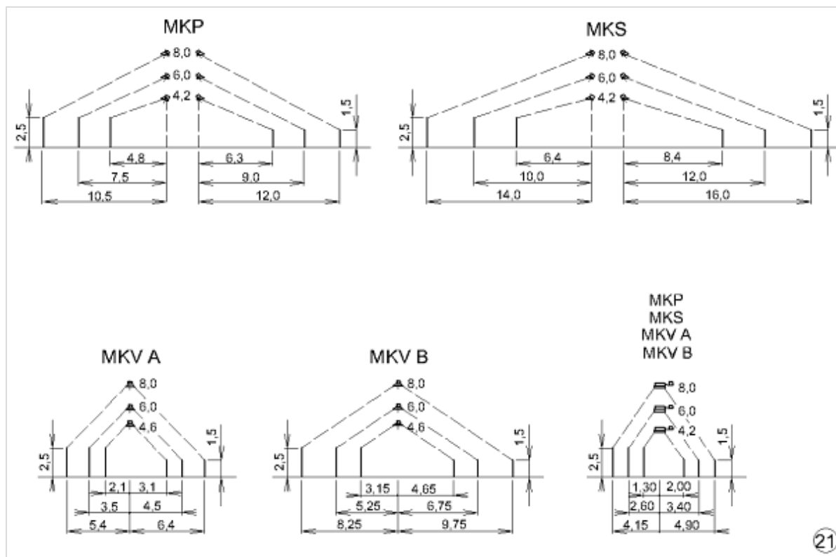
Obr. 21 - Dosah jednotlivých typů světelných zářičů při různých výškách zavěšení
